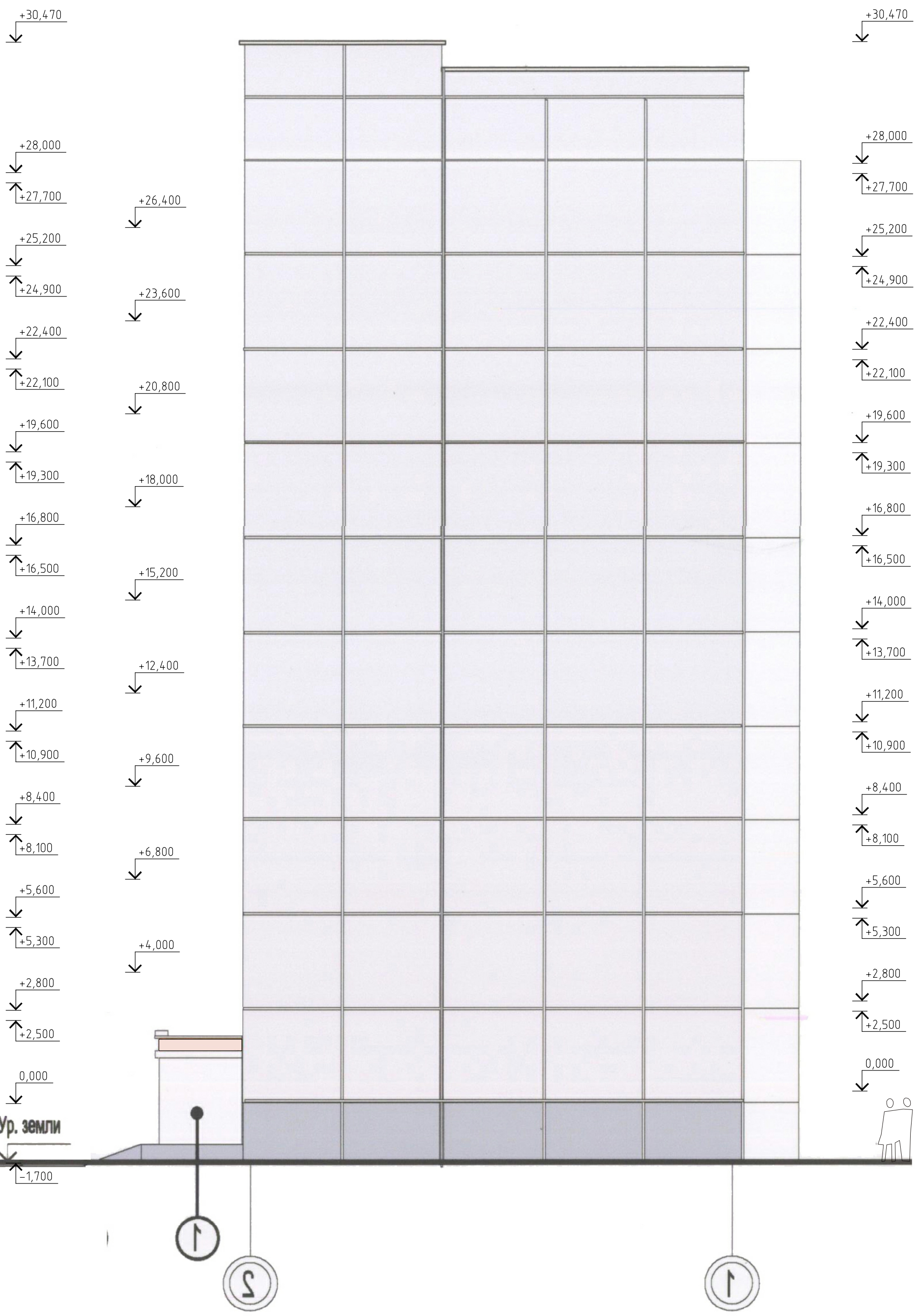
Чертеж торцевого юго-восточного фасада с цветовым решением в масштабе 1:100.
