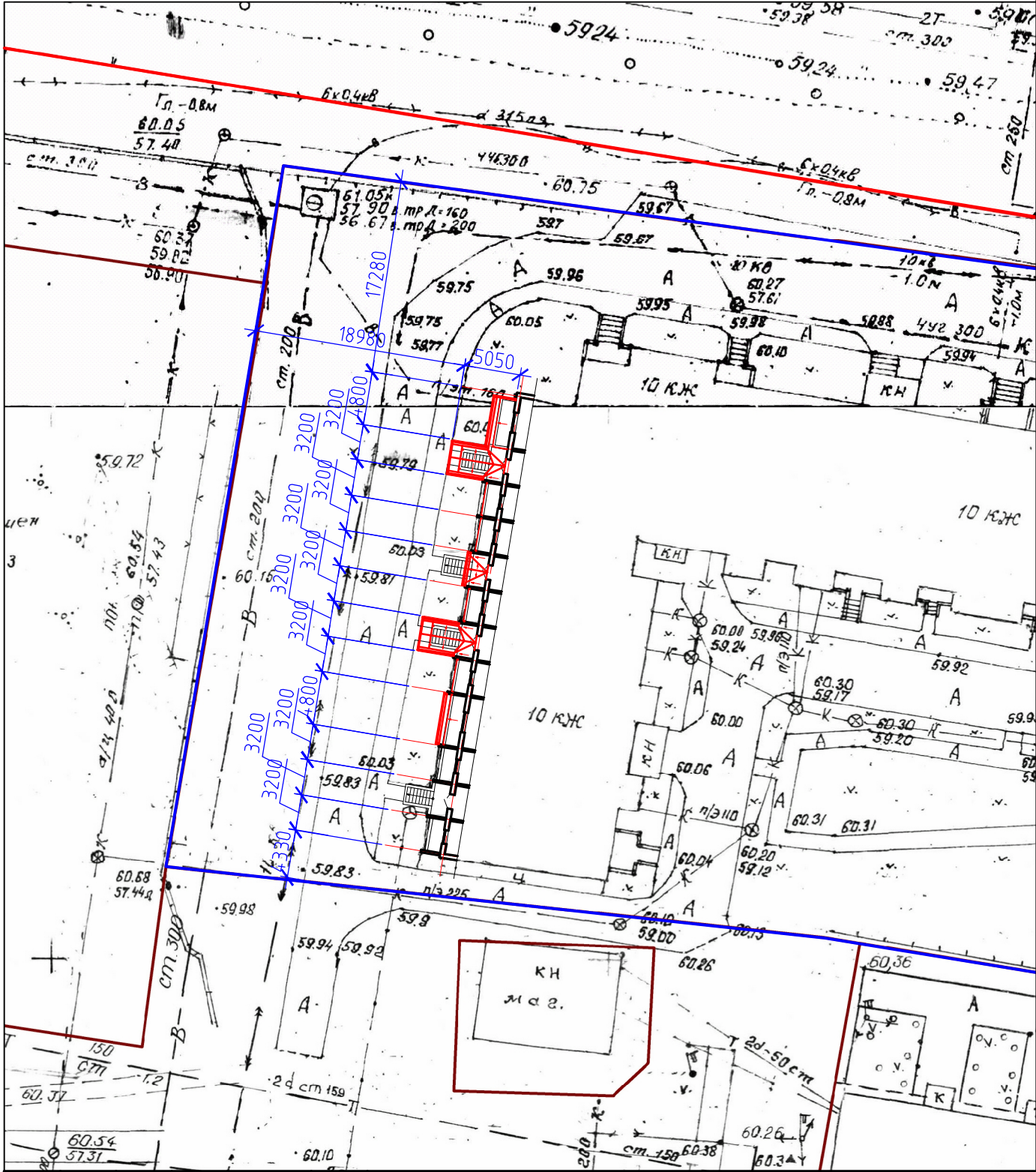
Разбивочный план в масштабе 1:500
