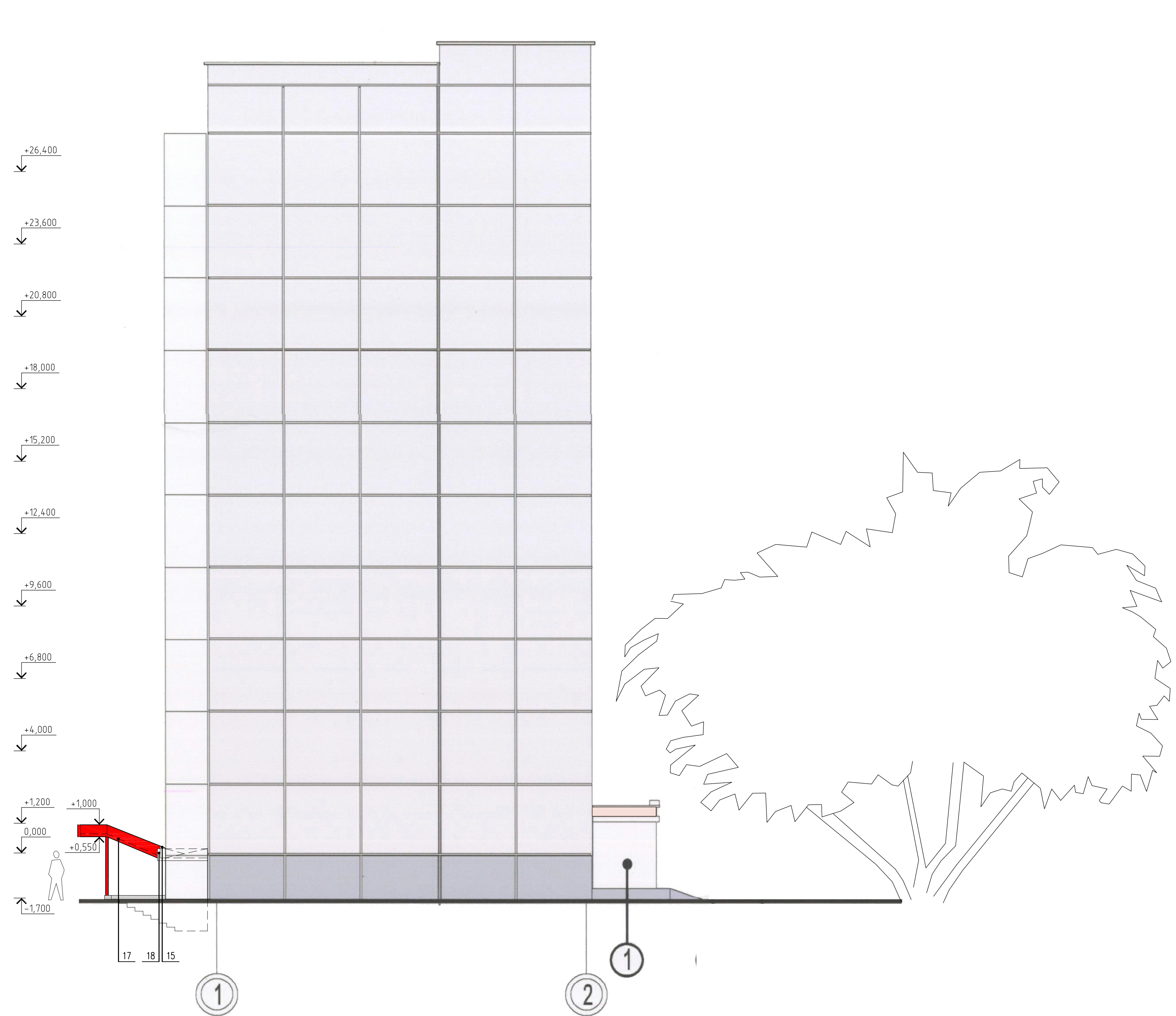
Чертеж торцевого юго-западного фасада с цветовым решением в масштабе 1:100.
