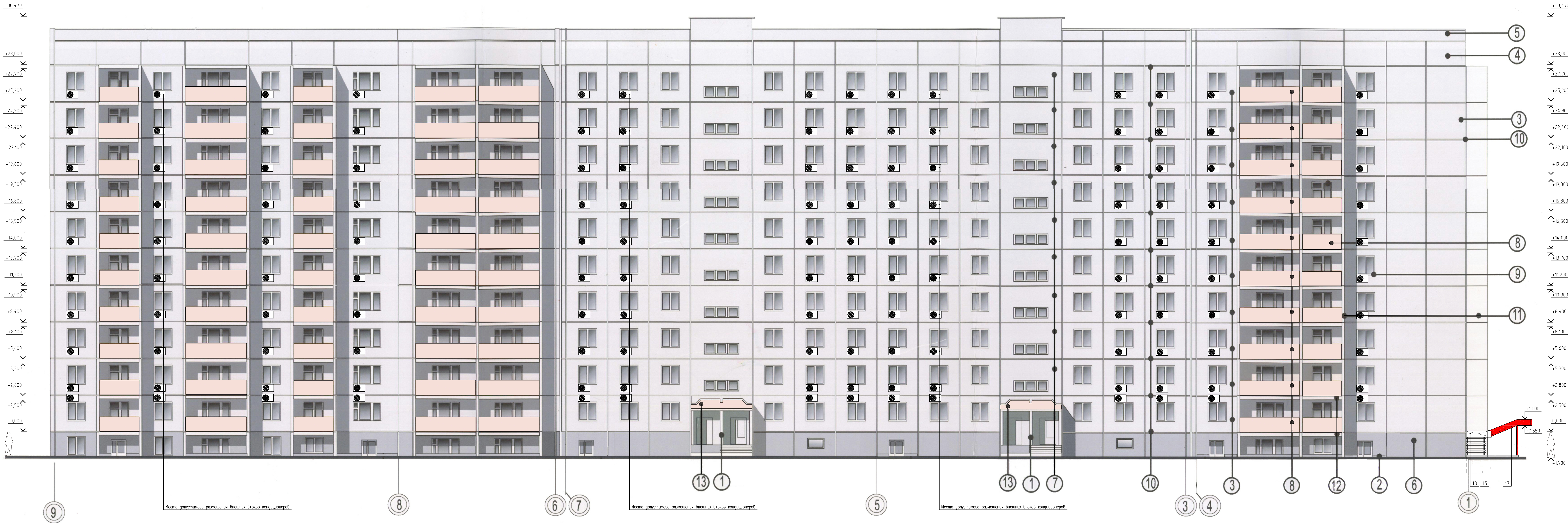
Чертеж дворового юго-западного фасада с цветовым решением в масштабе 1:100.
